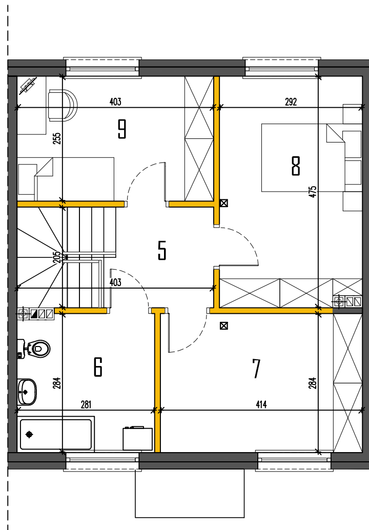
RZUT PIĘTRA
