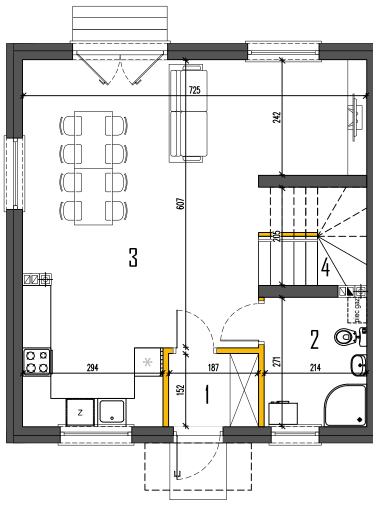
RZUT PARTERU
