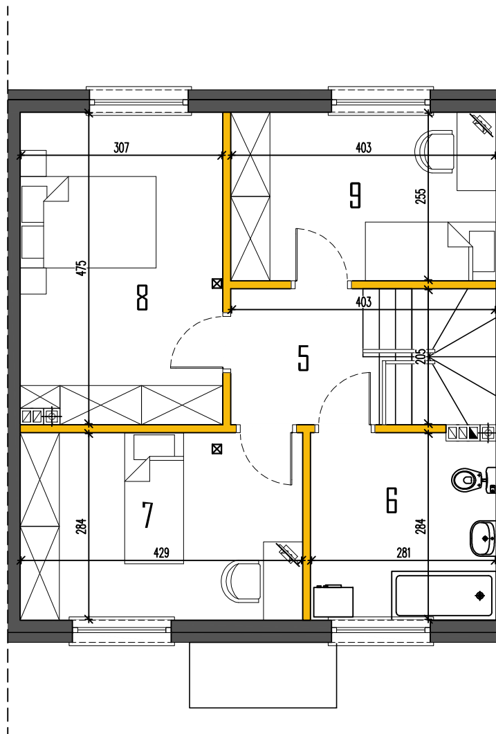
RZUT PIĘTRA
