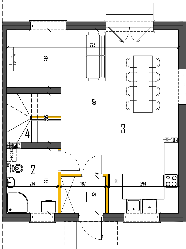
RZUT PARTERU
