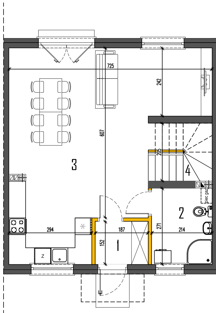
RZUT PARTERU
