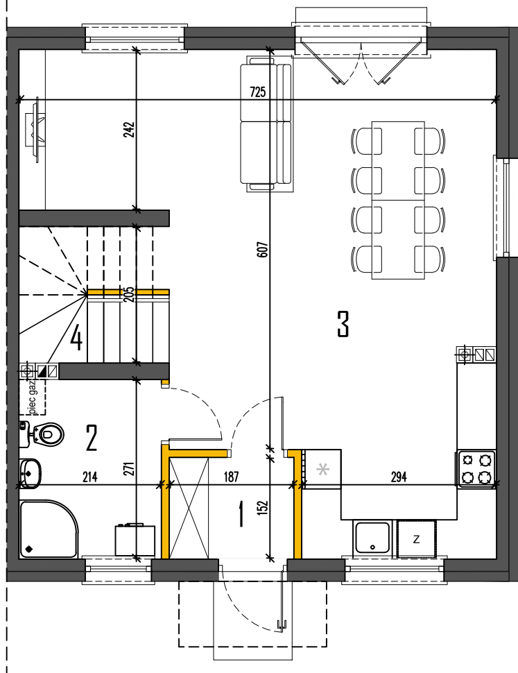
RZUT PARTERU
