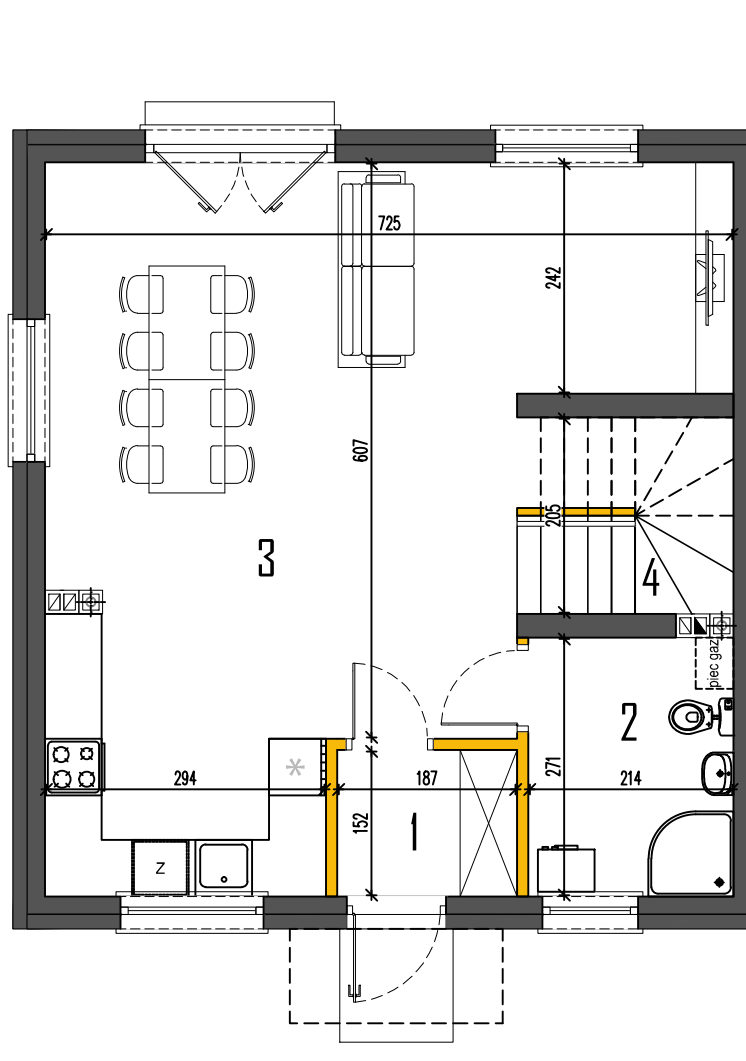
RZUT PARTERU
