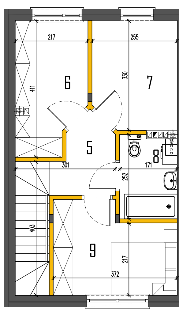
RZUT PIĘTRA
