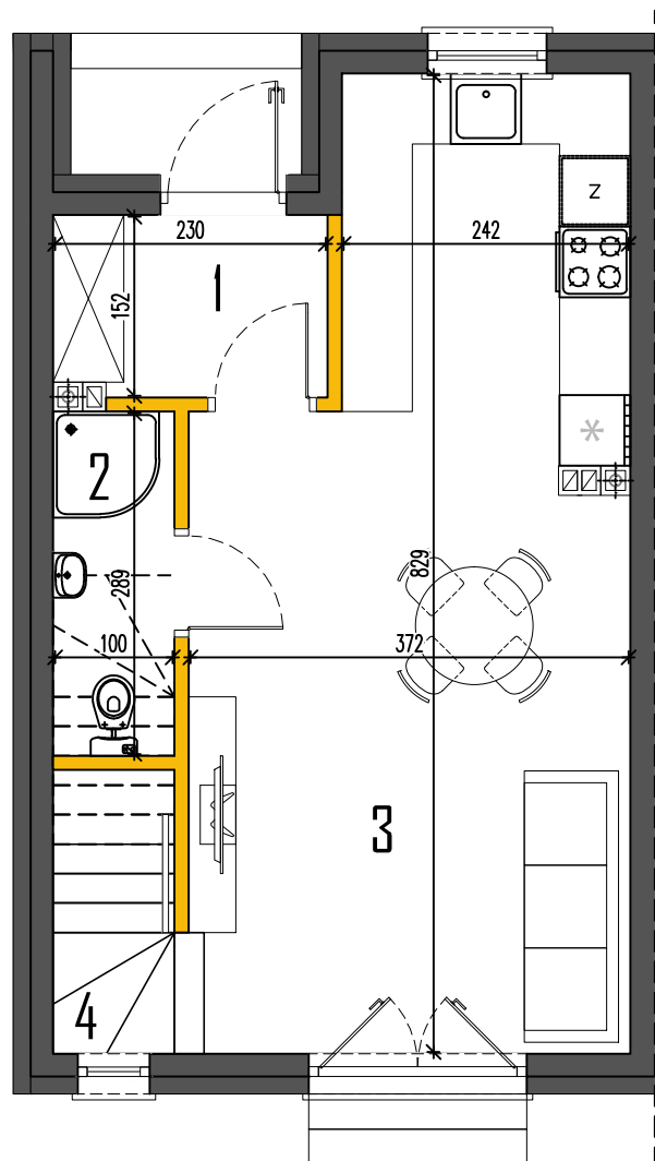
RZUT PARTERU
