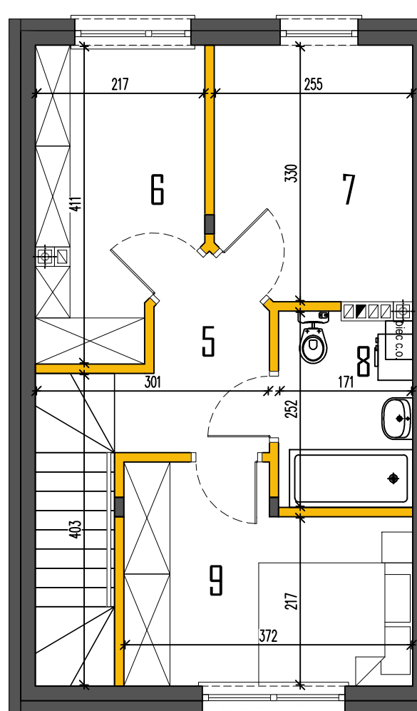
RZUT PIĘTRA
