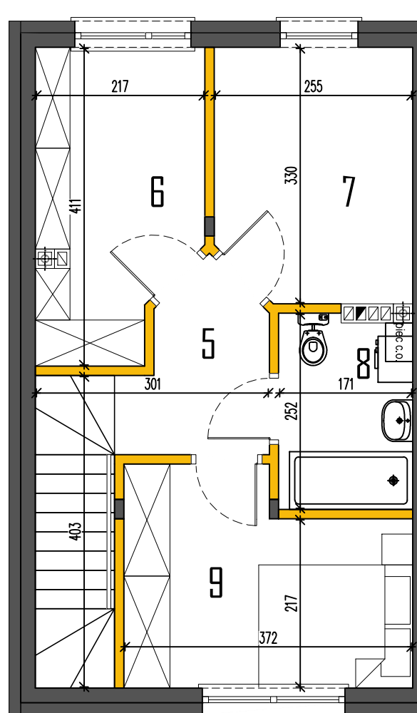
RZUT PIĘTRA
