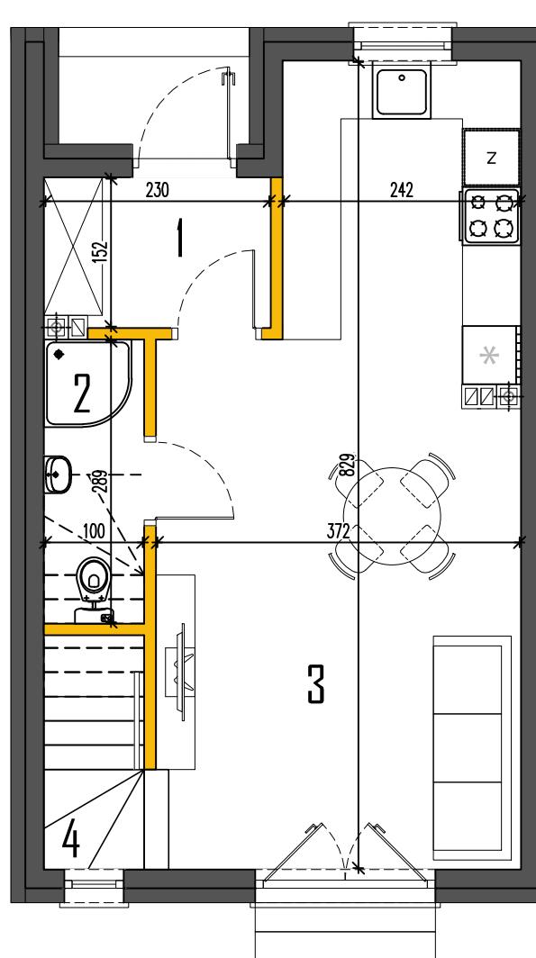
RZUT PARTERU
